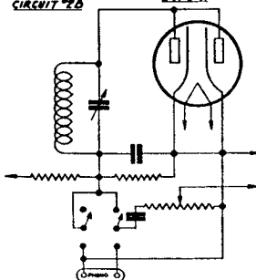
DET 6H6G
