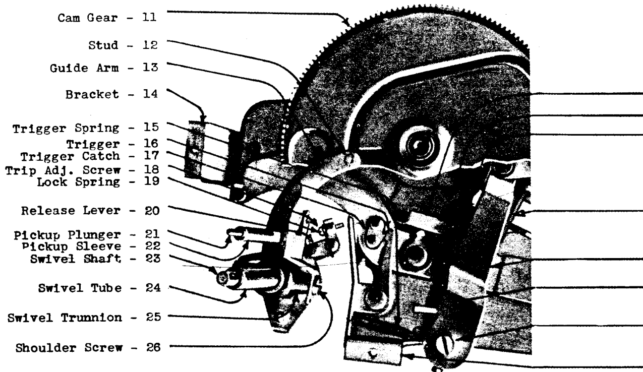
Sub-Plate A
