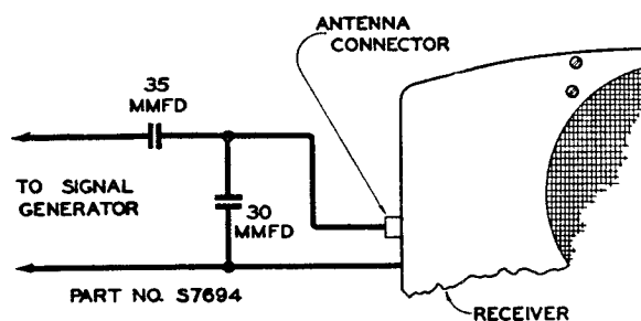
Fig. 3. Dummy Antenna
